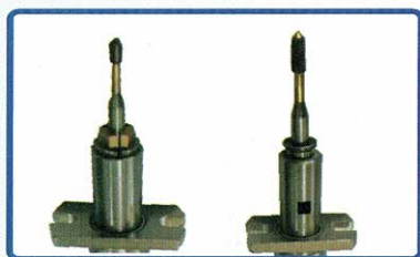
牙桿套組捍 Tap bar
